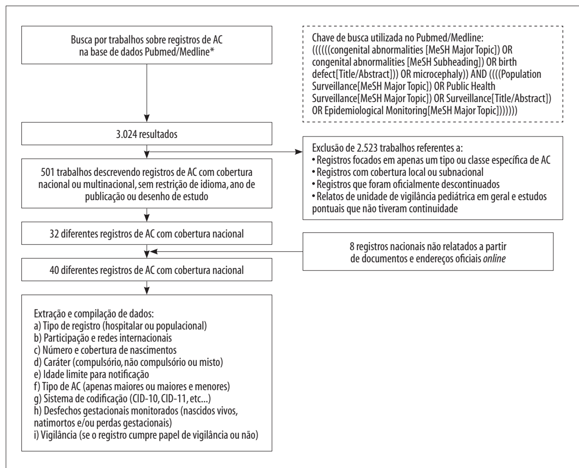
Figura 1 – Fluxograma das principais etapas metodológicas para a identificação e seleção de registros de anomalias congênicas com cobertura nacional existentes no mundo
