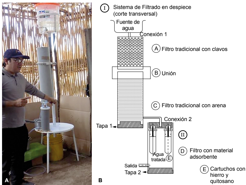
Figura 2. A. Instalación del filtro domiciliario; B. Esquema del sistema de filtración, compuesto por Filtro I, filtro tradicional de arena y virutas de hierro y Filtro II, material adsorbente de hierro cerovalente y quitosano.
