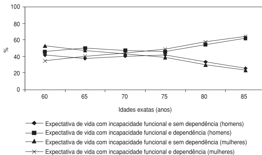
FIGURA 5. Proporção de anos a serem vividos com incapacidade funcional, decompostos de acordo com presença ou ausência de dependência, por sexo e idades exatas, Município de São Paulo (SP), Brasil, 2000 a
