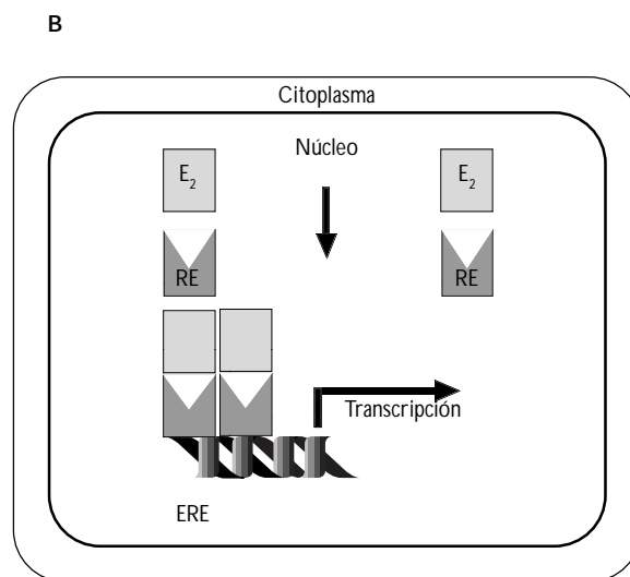
FIGURA 3. ESTRUCTURA QU6MICA (A) Y MECANISMO DE ACCIÓN DE LOS ANTIESTR6GENOS TIPO I (B). RE: RECEPTOR DE ESTRÓGENOS. ERE: ELEMENTO DE RESPUESTA A ESTRÓGENOS. AE: ANTIESTR6GENOS
