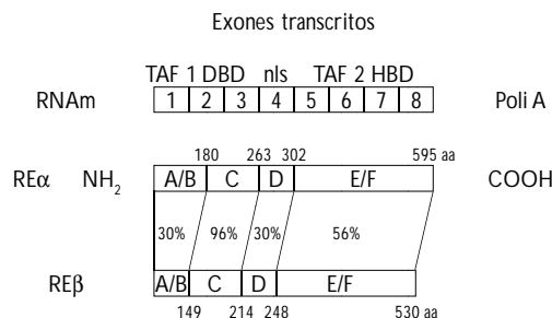
FIGURA 1. ESTRUCTURA DEL RECEPTOR DE ESTRÓGENOS. LOS NÚMEROS INTERIORES DEL RNAm CORRESPONDEN A LOS EXONES Y LAS LETRAS EXTERIORES A LAS REGIONES FUNCIONALES. EN LA PROTEÍNA, LAS LETRAS INTERIORES SEÑALAN LAS DIFERENTES REGIONES DEL RECEPTOR Y LOS NÚMEROS EXTERIORES CORRESPONDEN AL NÚMERO DE AMINOÁCIDOS (AA). LOS PORCENTAJES REPRESENTAN EL GRADO DE HOMOLOGÍA ENTRE LOS DOMINIOS DE LAS DOS ISOFORMAS DE RE (MODIFICADO POR OGAWA, 1998). TAF 1 y 2 : DOMINIO DE ACTIVACIÓN TRANSCRIPCIONAL. DBD : DOMINIO DE UNIÓN AL DNA. NLS : SEÑAL DE LOCALIZACIÓN NUCLEAR. HBD : DOMINIO DE UNIÓN A LA HORMONA
