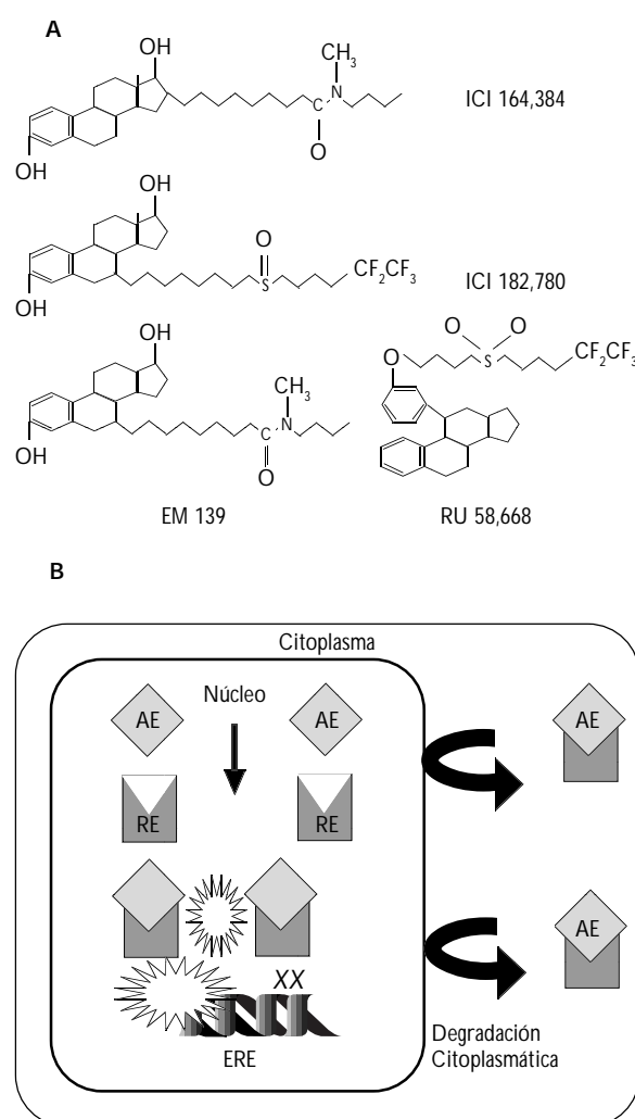
FIGURA 4. ESTRUCTURA QU3MICA (A) Y MECANISMO DE ACCI3N DE LOS ANTIESTR6GENOS TIPO II (B). RE: RECEPTOR DE ESTR6GENOS. ERE: ELEMENTO DE RESPUESTA A ESTR6GENOS. AE: ANTIESTR6GENOS
