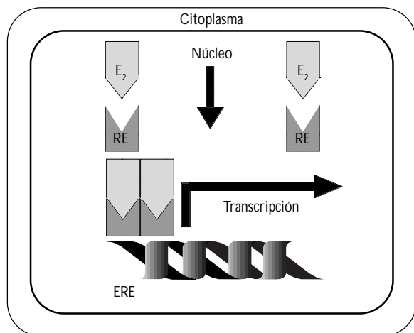
FIGURA 2. MODELO DEL MECANISMO DE ACCIÓN DEL ESTRADIOL. E 2 : ESTRADIOL. RE: RECEPTOR DE ESTRÓGENOS. ERE: ELEMENTO DE RESPUESTA A ESTRÓGENOS
