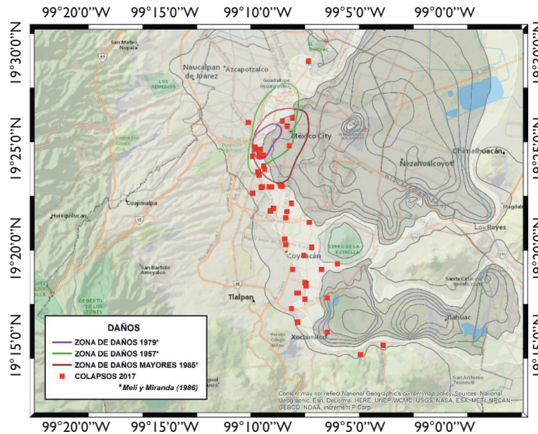
FIGURA 6. COLAPSOS OCURRIDOS POR EL SISMO DEL 19 DE SEPTIEMBRE DE 2017 Y LAS ZONAS DE DAÑOS GENERADOS POR LOS SISMOS DE 1957, 1979 Y 1985, REPORTADOS POR MELI Y MIRANDA 5
