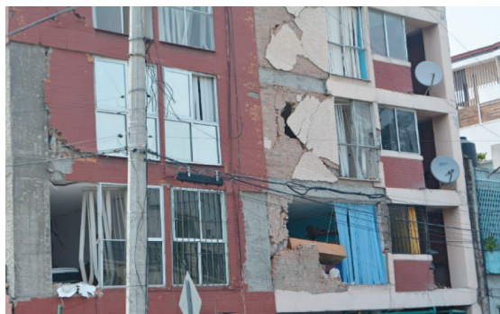
Muros no estructurales (Ing. Francisco García Jarque)
