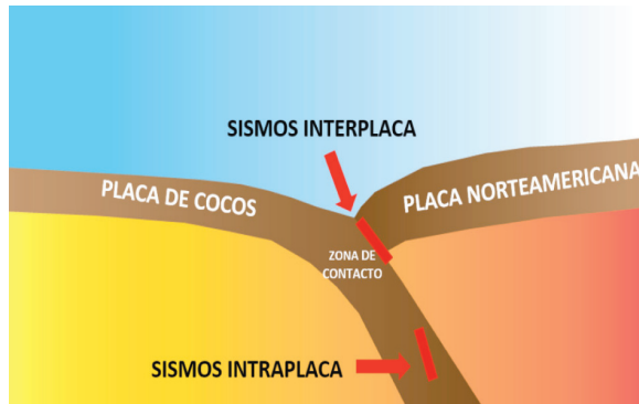
FIGURA 3. ESQUEMA DE LOS SISMOS DE SUBDUCCIÓN DE INTERPLACA Y LOS SISMOS INTRAPLACA
